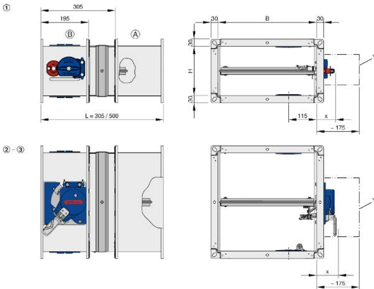
Bild 2: FKA2-EU med smältsäkring
