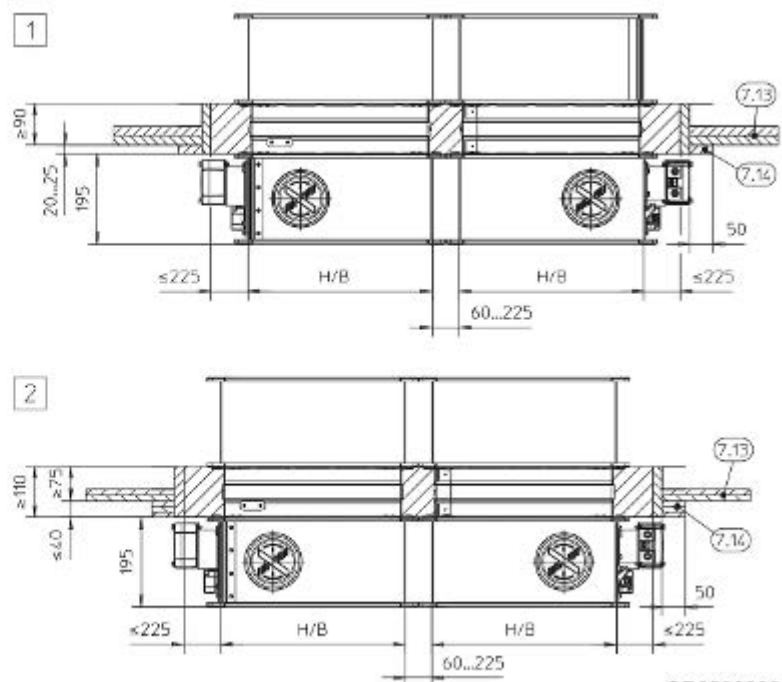
Bild 123: Murbruksbaserad installation i schaktvägg, fläns mot fläns, illustration visar montering sida vid sida (gäller även montering av spjäll ovanför varandra)
