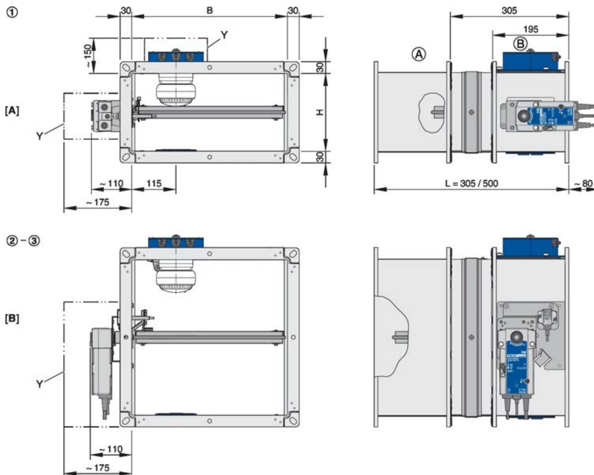
Bild 7: FKA2-EU med Belimo fjäderåtergångsmotor och kanlrökdetect
