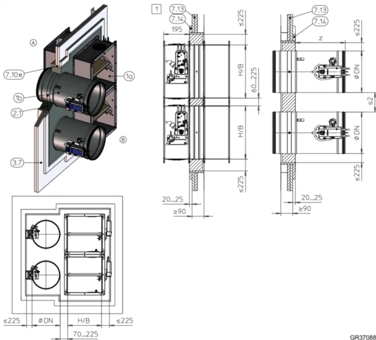
Bild 125: Murbruksbaserad installation i schaktvägg, FKA2-EU och FKR-EU kombinerat
