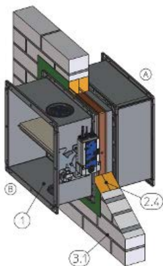
Bild 61: Torr installation utan murbruk med brandskiva i massiv vägg
