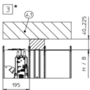
Bild 96: Murbruksbaserad installation i en lätt skiljevägg, korsvirkeskonstruktion
