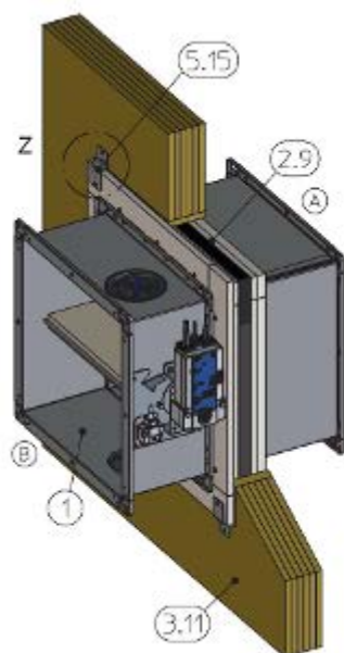
Bild 117: Torr installation utan murbruk i en massiv trävägg eller korslaminerad trävägg (CLT), med installationskit ES
