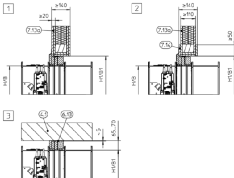
Bild 106: Torka installation utan murbruk i korsvirkeskonstruktion, med installationskit ES
