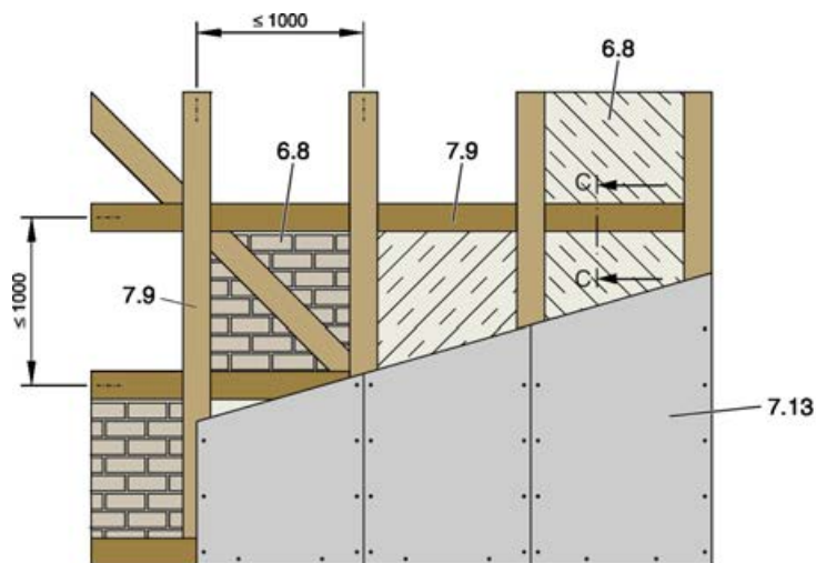
Bild 91: Lätt skiljevägg, korsvirkeskonstruktion med beklädnad på båda sidor
