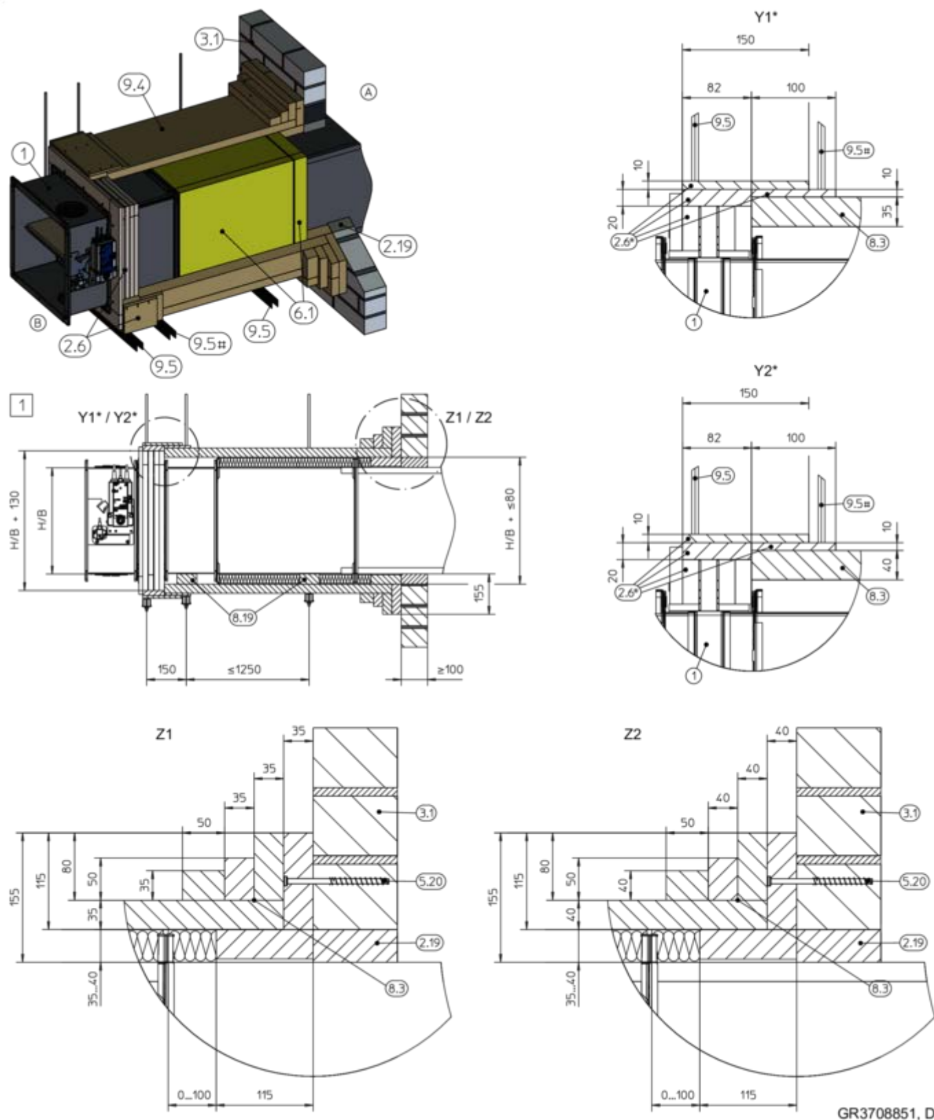
Bild 57: Torr installation utan murbruk på avstånd från massiva väggar med installationskit WE (vägganslutet)
