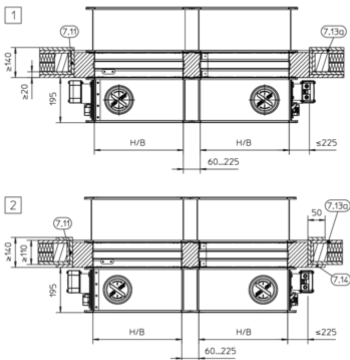
Bild 97: Murbruksbaserad installation i en lätt skiljevägg, korsvirkeskonstruktion, fläns mot fläns, illustration visar montering sida vid sida (gäller även montering av spjäll ovanför varandra)
