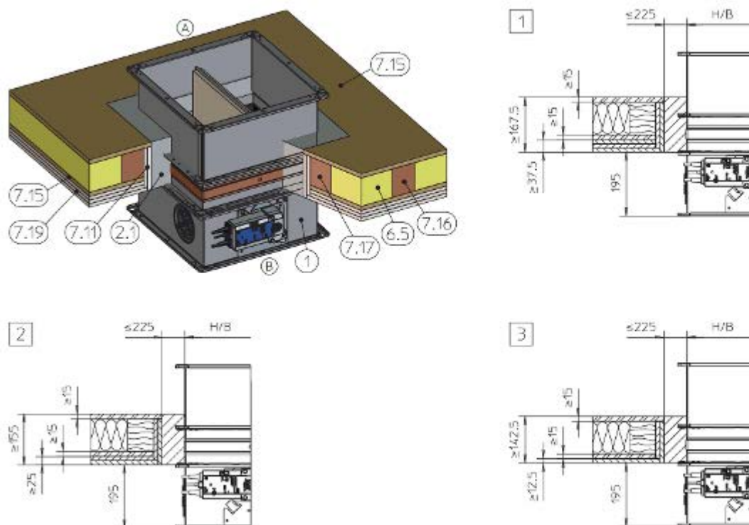
Bild 154: Murbruksbaserad installation i tak med träbjälkar / limträtak, nedhängt (illustrationen är ett exempel; andra takkonstruktioner kan vara möjliga på begäran)
