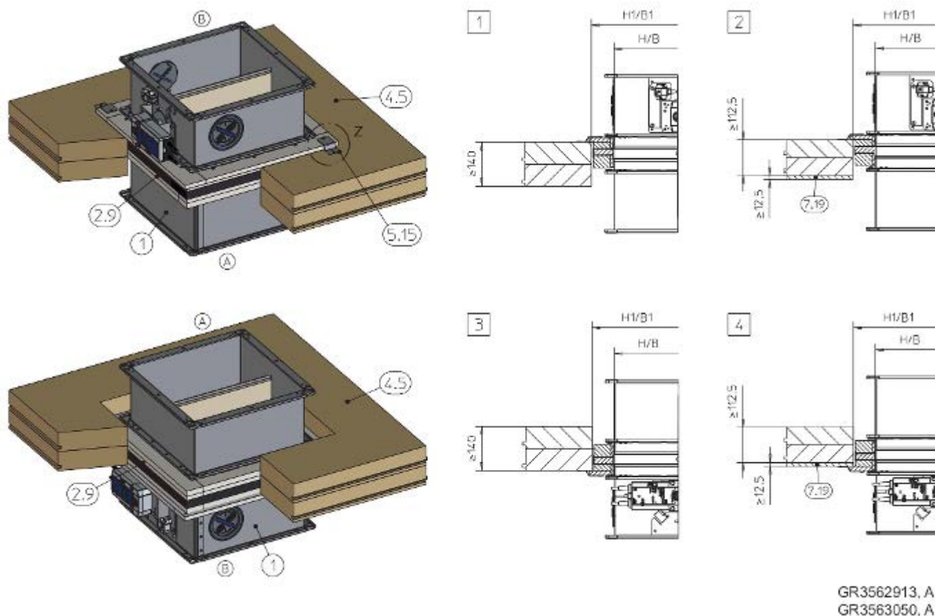
Bild 152: Torr installation utan murbruk med installationskit ES i massivt trätak, stående och nedhängd
