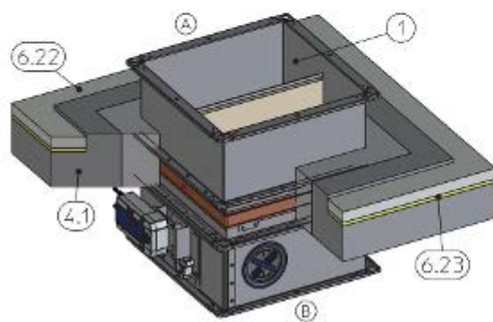
Bild 131: Murbruksbaserad installation i en massiv våningsavskiljning med golv- och fotljudsisolering, nedhängd eller stående
