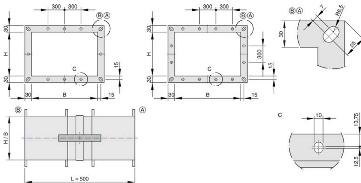
Bild 4: Flänshål L = 500 mm – ojämnt och jämnt antal hål
