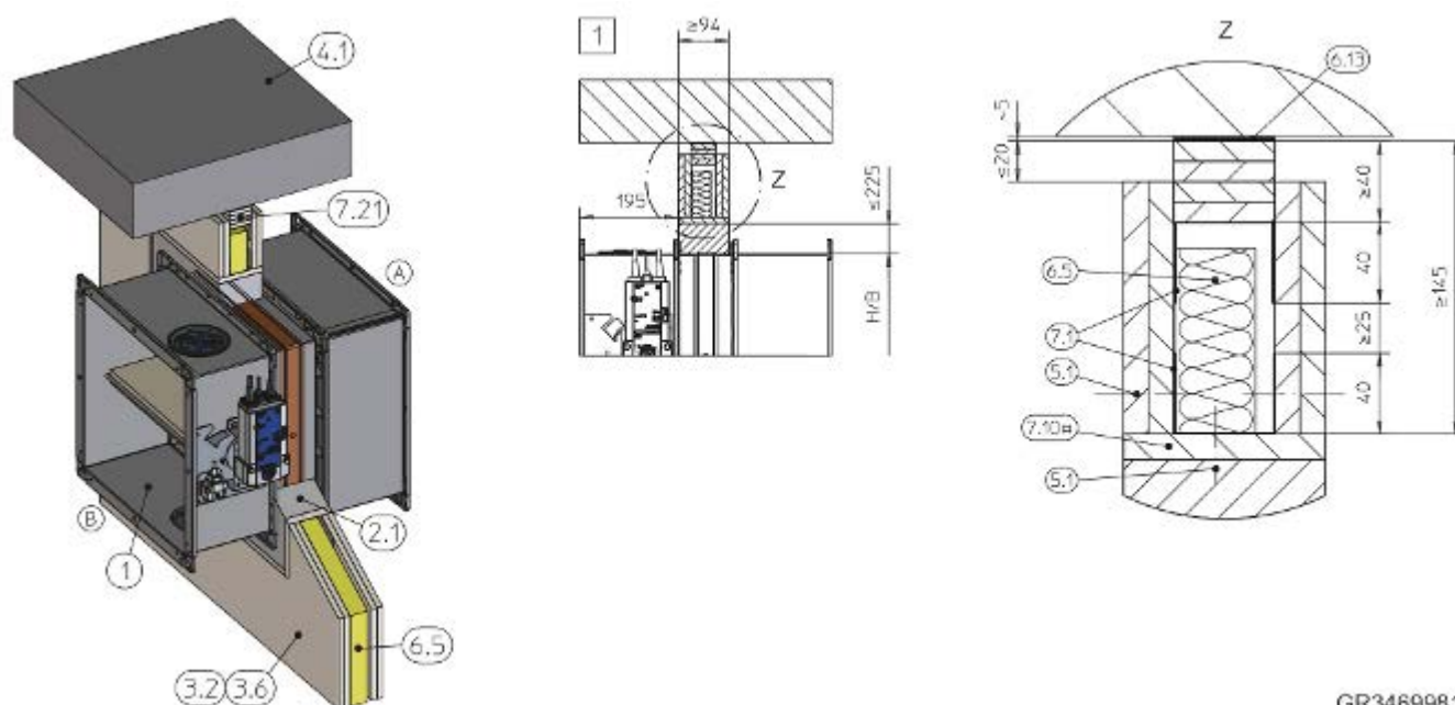
Bild 74: Murbruksbaserad installation i en lätt skiljevägg, under en flexibel takfog
