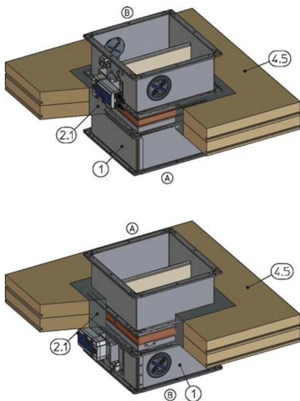
Bild 151: Murbruksbaserad installation i massivt trätak, nedhängd eller stående
