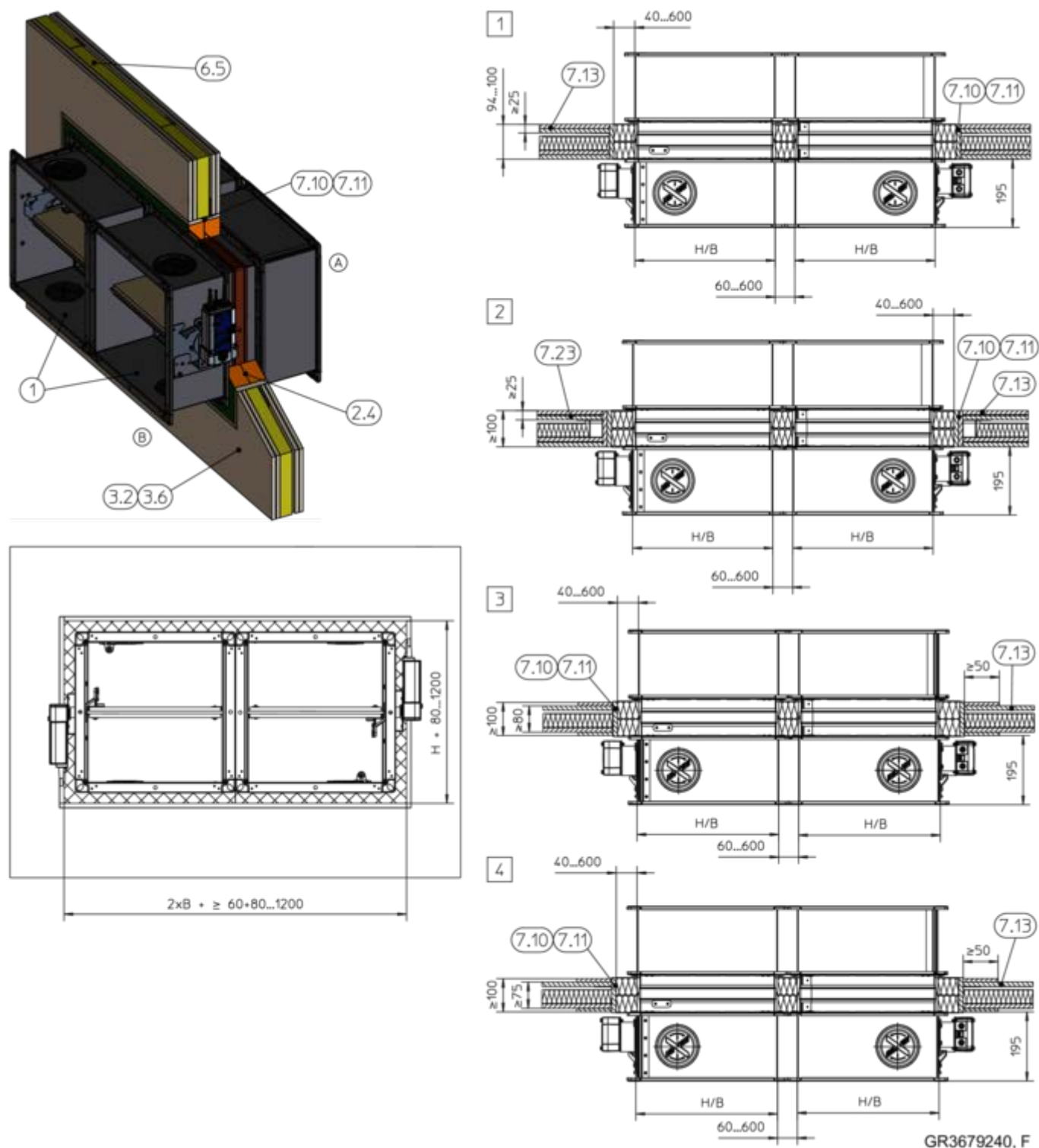
Bild 87: Torr installation utan murbruk i en lätt skiljevägg, med en brandskiva, fläns mot fläns, illustrationen visar montering sida vid sida (gäller även montering av spjäll ovanför varandra)
