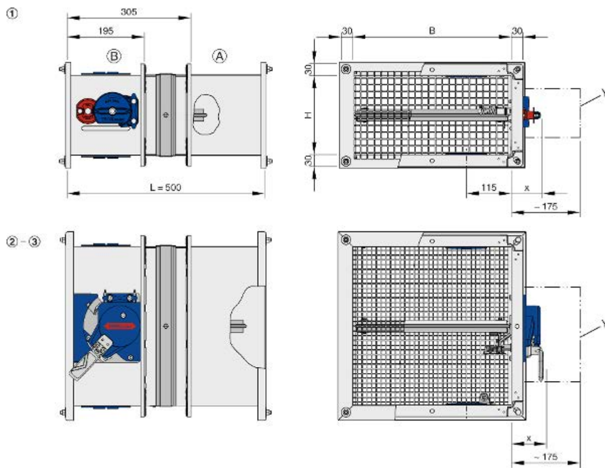
Bild 8: FKA2-EU med smältsäkring och skyddsgaller som överlufts-enhet
