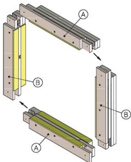
Bild 35: Installationskit WA för torr installation utan murbruk - montering
