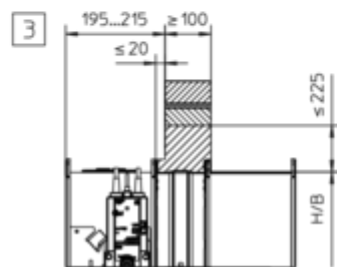
Bild 46: Murbruksbaserad installation i en massiv vägg
