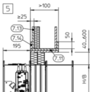
Bild 86: Torr installation utan murbruk i en lätt skiljevägg, med en brandskiva
