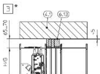
Bild 117: Torr installation utan murbruk i en massiv trävägg eller korslaminerad trävägg (CLT), med installationskit ES
