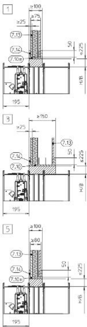
Bild 70: Murbruksbaserad installation i en lätt skiljevägg
