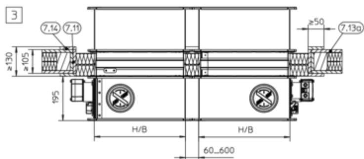
Bild 110: Torr installation utan murbruk i en lätt skiljevägg med träregel, med en brandskiva, fläns mot fläns, illustrationen visar montering sida vid sida (gäller även montering av spjäll ovanför varandra)
