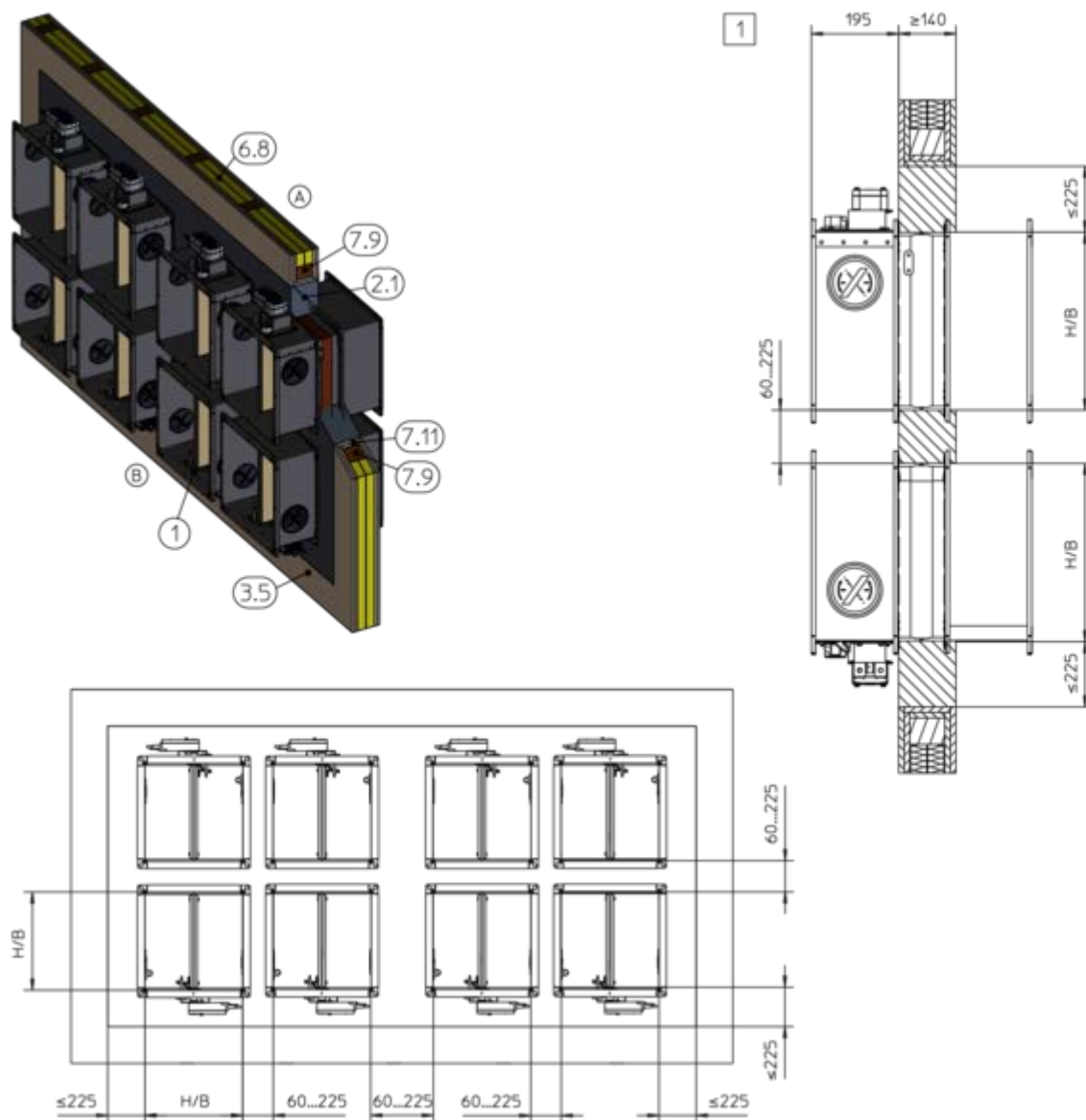
Bild 102: Murbruksbaserad installation – flera enheter i en installationsöppning i korsvirkeskonstruktion
