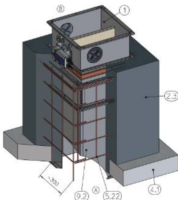
Bild 137: Murbruksbaserad installation med betongfundament i en massiv våningsavskiljning, upprätt
