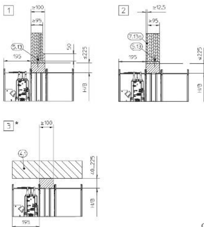
Bild 116: Murbruksbaserad installation i en massiv trävägg eller korslaminerade trävägg (CLT)
