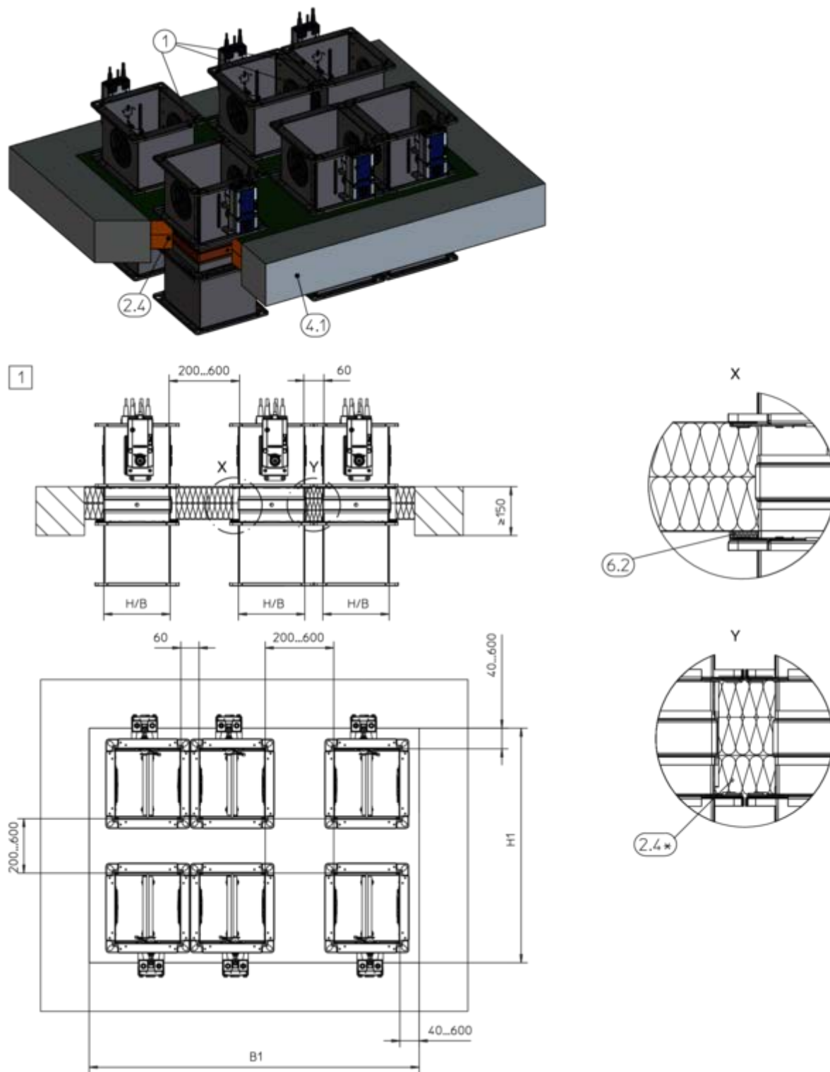
Bild 150: Torr installation utan murbruk med brandskiva i massiv våningsavskiljning, flera enheter, fläns mot fläns, illustration visar stående installation (gäller även nedhängd installation)
