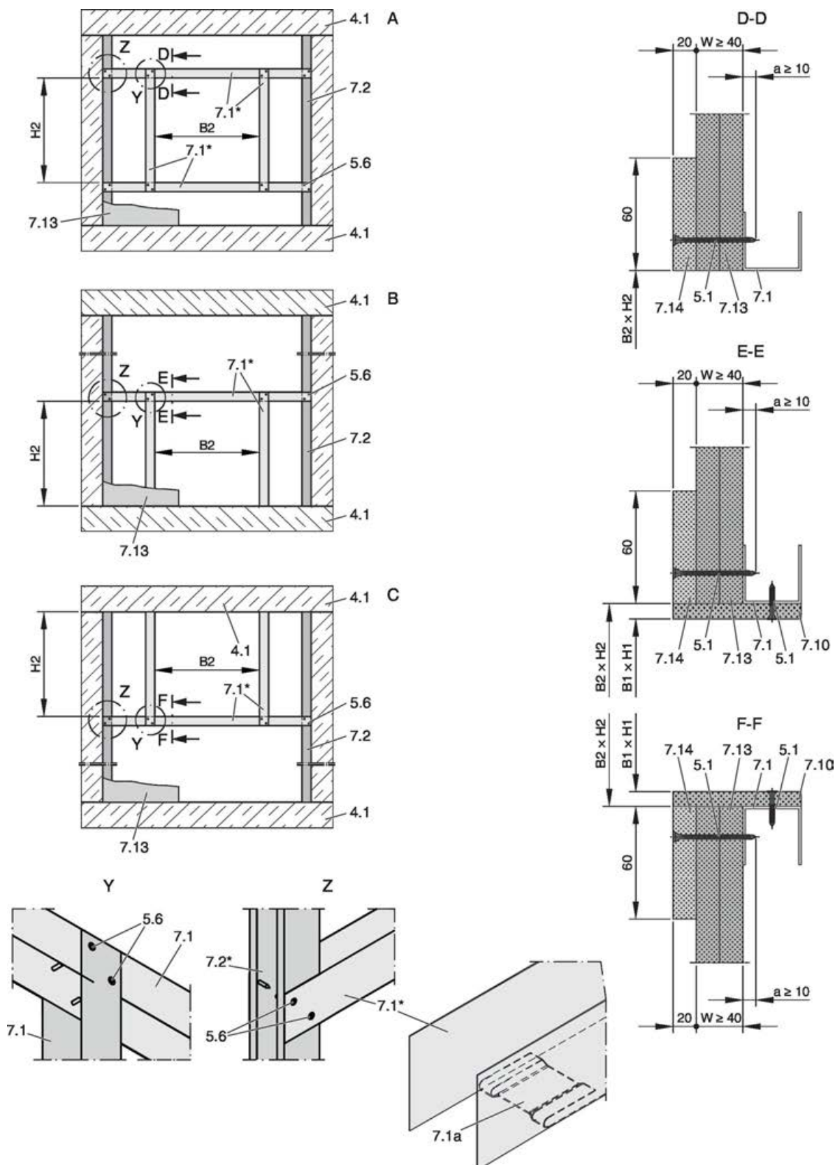
Bild 127: Schaktvägg utan metallreglar och beklädnad på en sida
