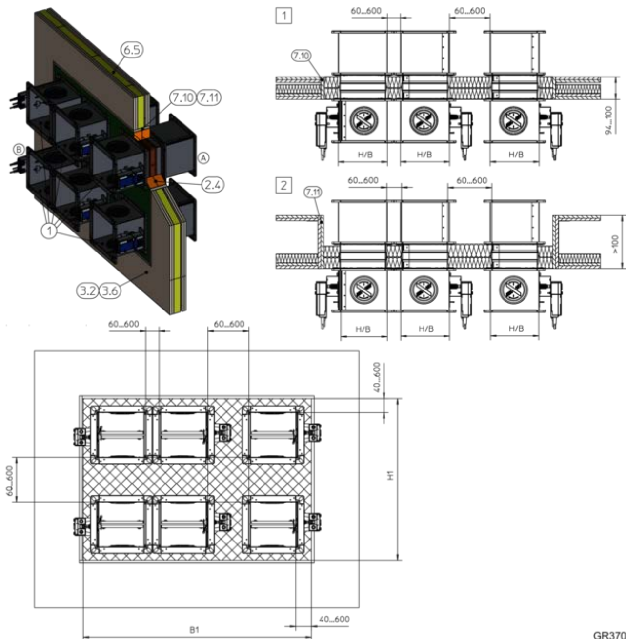
Bild 88: Torr installation utan murbruk i en lätt skiljevägg, med en brandskiva, fläns mot fläns, flera enheter, illustrationen visar montering sida vid sida (gäller även montering av spjäll ovanför varandra)
