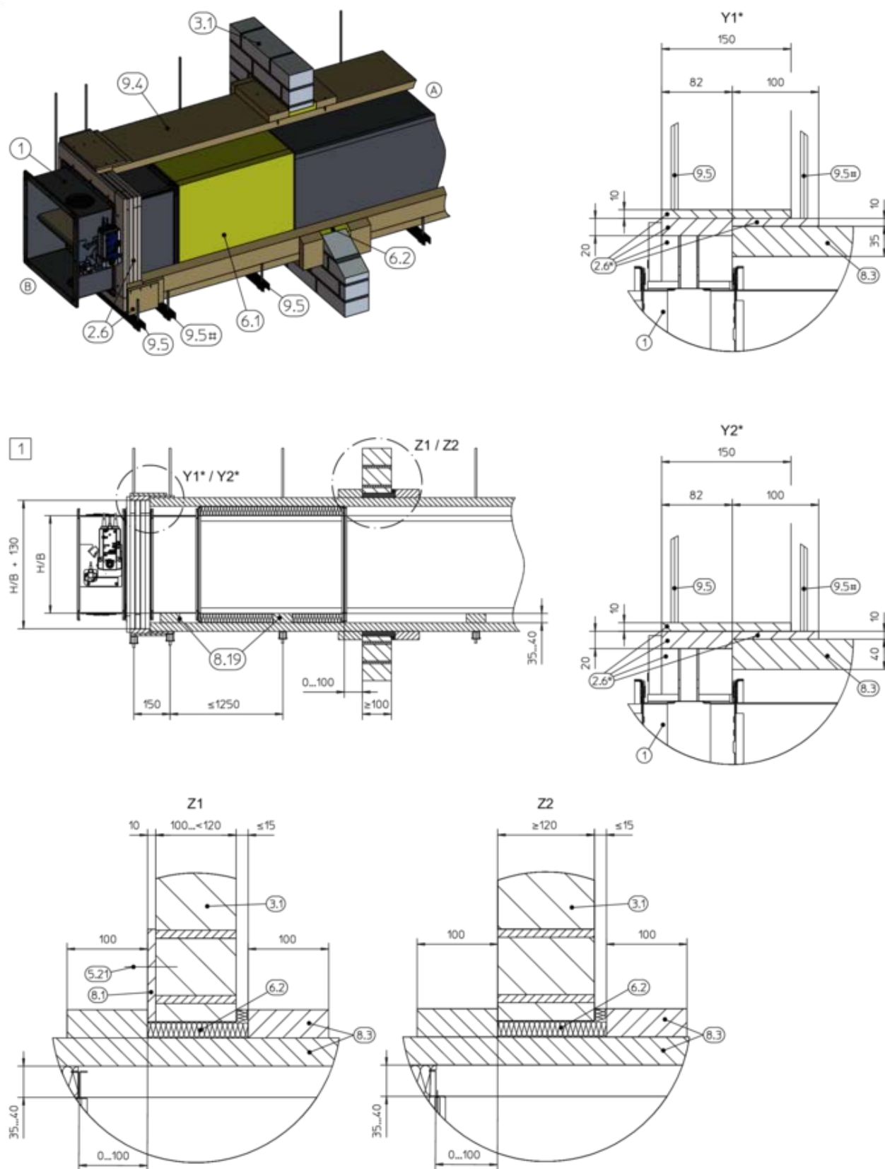
Bild 59: Torr installation utan murbruk på avstånd från massiva väggar med installationskit WE (väggenomföring)
