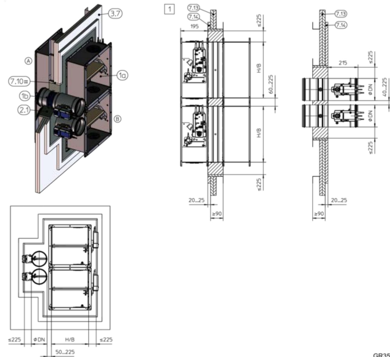
Bild 124: Murbruksbaserad installation i schaktvägg, FKA2-EU och FKRS-EU kombinerat
