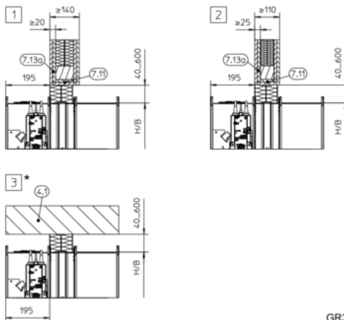
Bild 111: Torr installation utan murbruk i korsvirkeskonstruktion, med brandskiva
