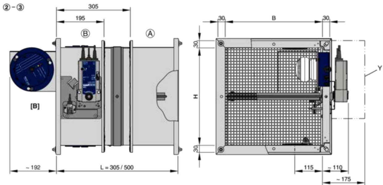
Bild 10: FKA2-EU med fjäderåtergångsmotor och kanalrökdetektor som överluftspjäll – variant med fäste på drivsidan uppe till höger (visas för storlek 2 och 3)
