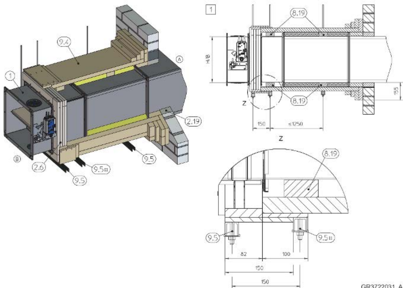
Bild 158: Torr installation utan murbruk med installationskit WE
