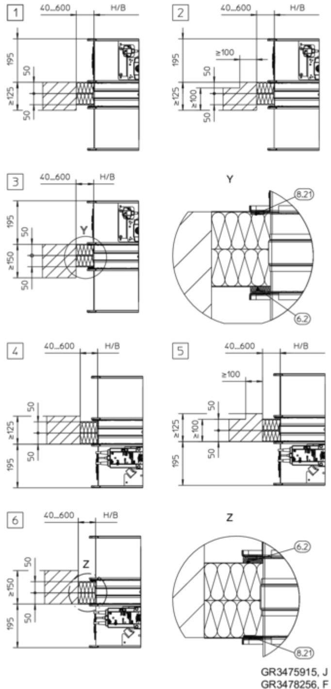
Bild 148: Torr installation utan murbruk i massiv våningsavskiljning, med brandskiva, stående och nedhängd
