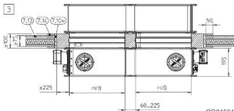
Bild 71: Murbruksbaserad installation i en lätt skiljevägg, fläns mot fläns, illustration visar montering sida vid sida (gäller även montering av spjäll ovanpå varandra)
