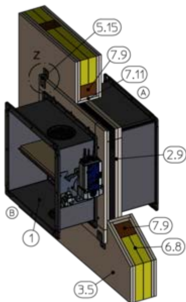
Bild 106: Torka installation utan murbruk i korsvirkeskonstruktion, med installationskit ES
