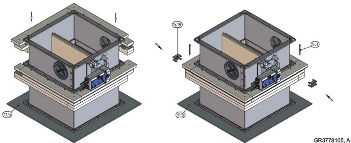
Bild 36: Installationskit WA för torr installation utan murbuk - montering
