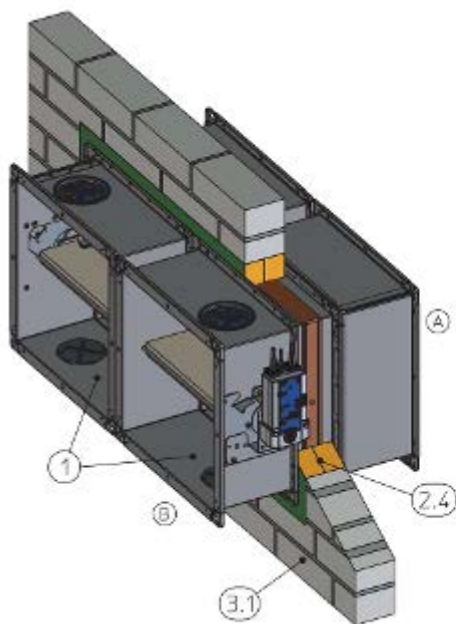
Bild 62: Torr installation utan murbruk i en massiv vägg, med brandskiva, fläns mot fläns, illustration visar montering sida vid sida (gäller även montering av spjäll ovanpå varandra)
