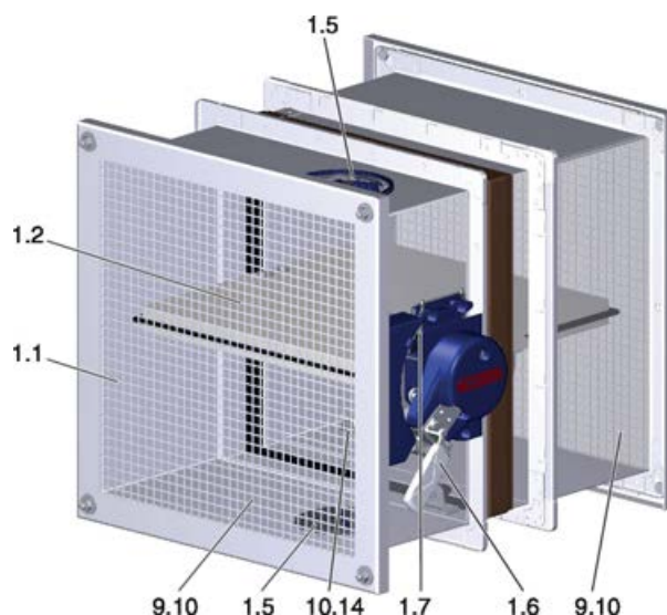
Bild 14: FKA2-EU med smältsäkring och skyddsgaller som överluftsenhet
