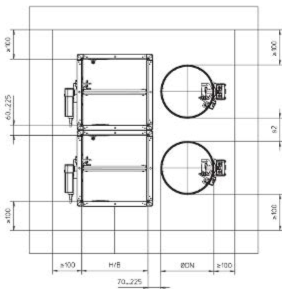
Bild 139: Murbruksbaserad installation med betongfundament i en massiv våningsavskiljning, stående, FKA2-EU och FKR-EU kombinerat
