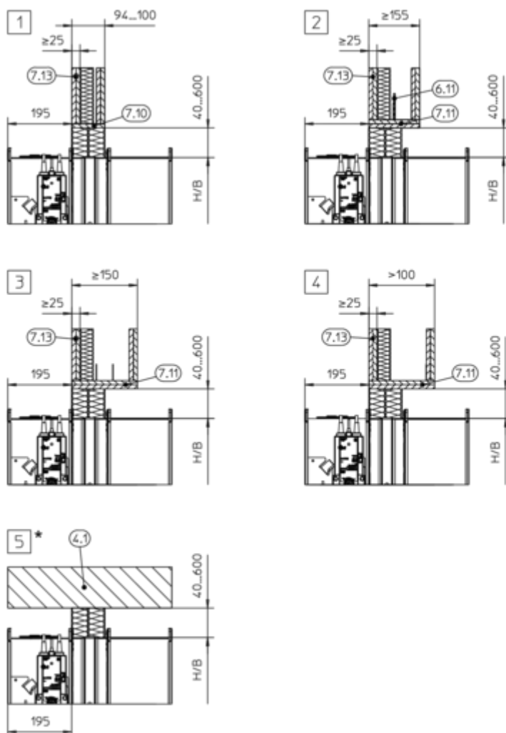
Bild 85: Torr installation utan murbruk i en lätt skiljevägg, med en brandskiva
