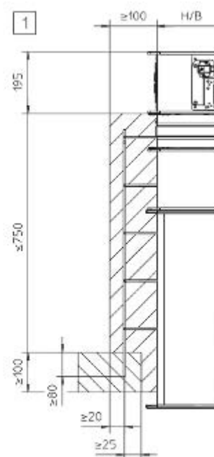
Bild 137: Murbruksbaserad installation med betongfundament i en massiv våningsavskiljning, upprätt
