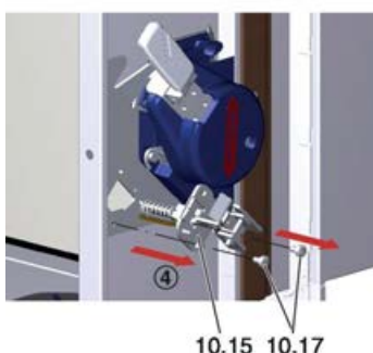
Bild 182: Ta bort smältsäkringens hållare
