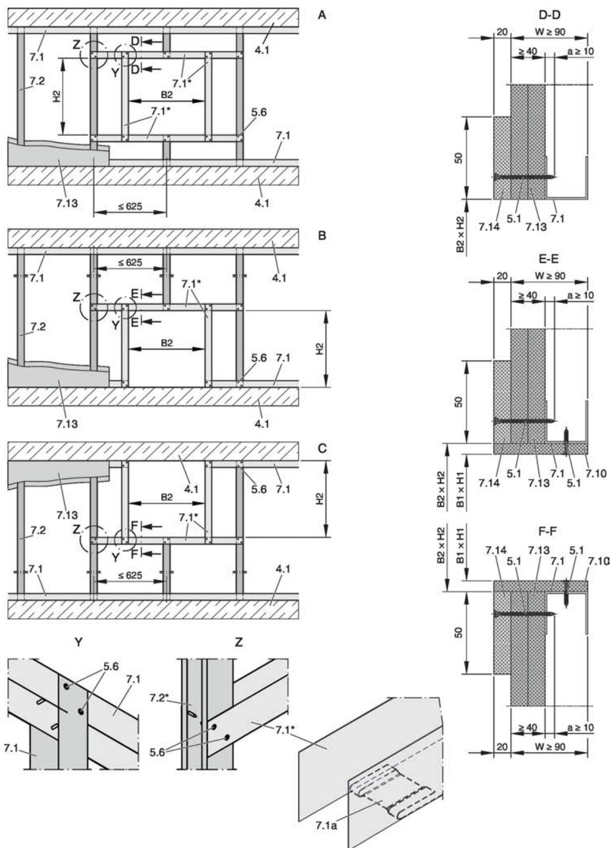
Bild 121: Schaktvägg med metallreglar och beklädnad på ena sidan (detaljvyer visas med W = 90 \text{ mm} )
